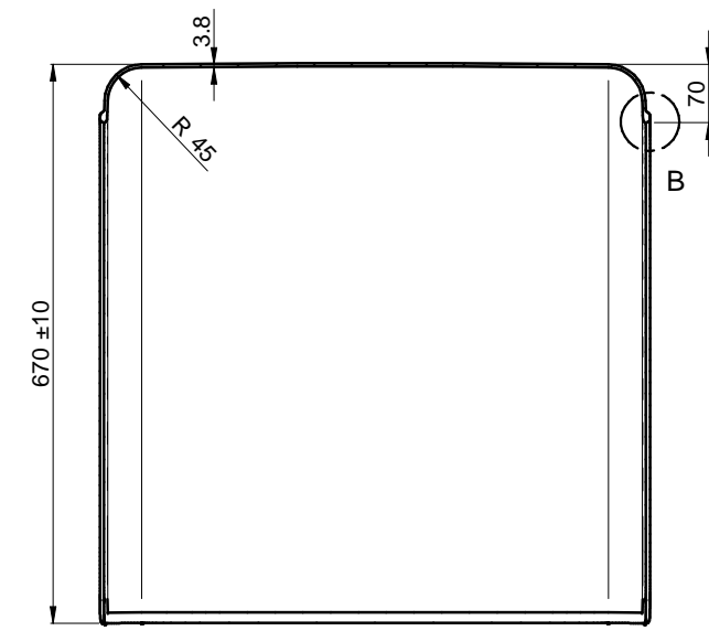
SEZIONE A-A
