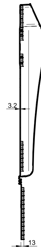
SEZIONE A-A
