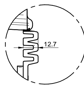
DETTAGLIO C
