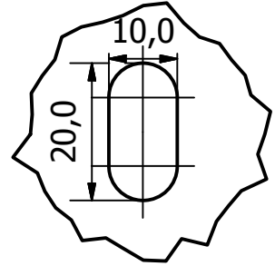
DETAIL A ( 1 : 1 ) TYP 6 PLACES
